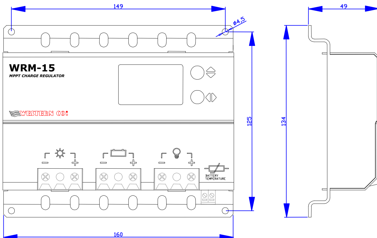
Fig. 8 Dimensions
